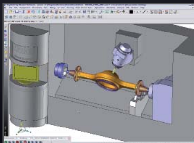
Fraisage 4&5 axes positionnés.
